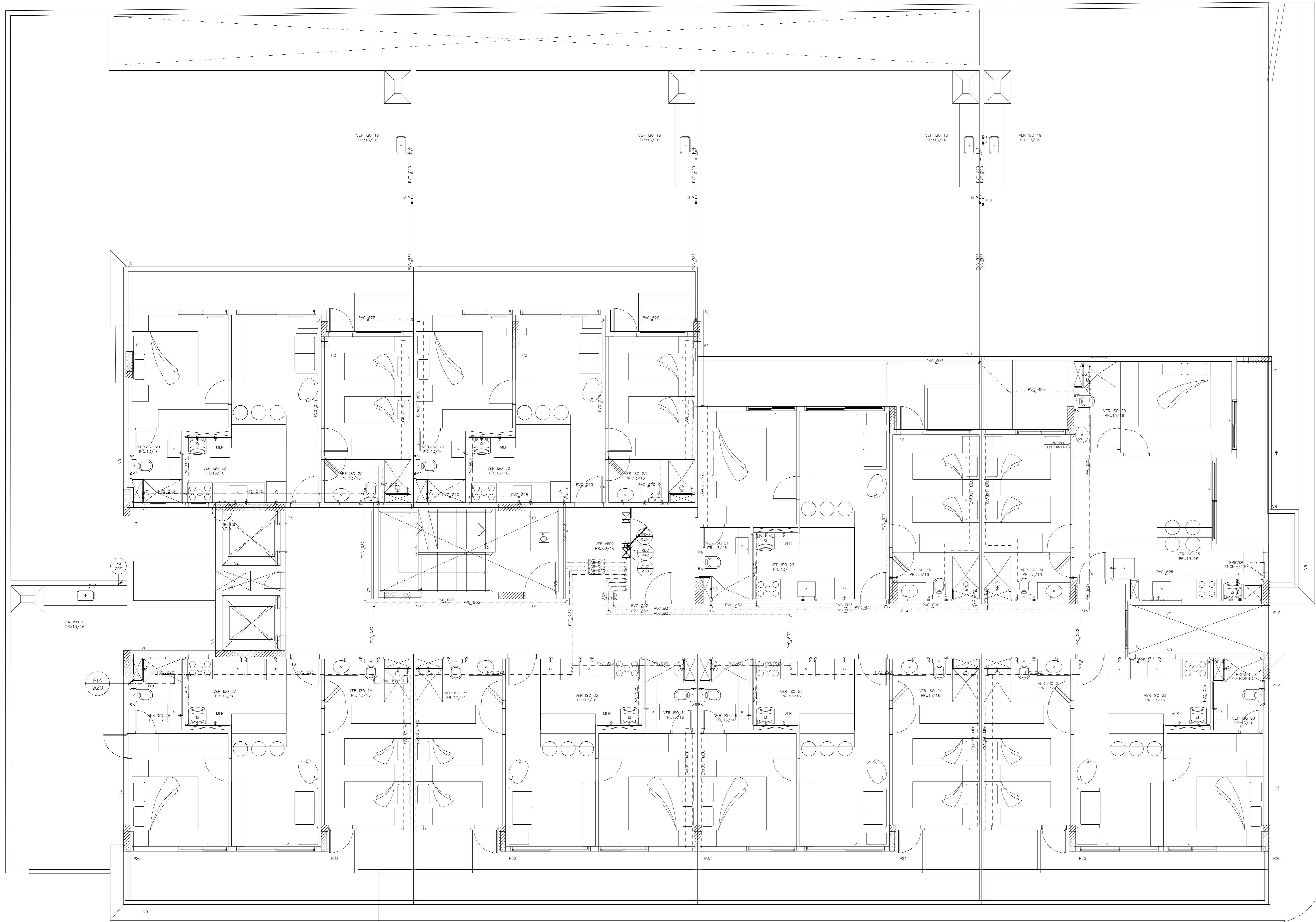
PLANTA BAIXA - 2º PAVIMENTO ÁGUA FRIA ESC.: 1:50
